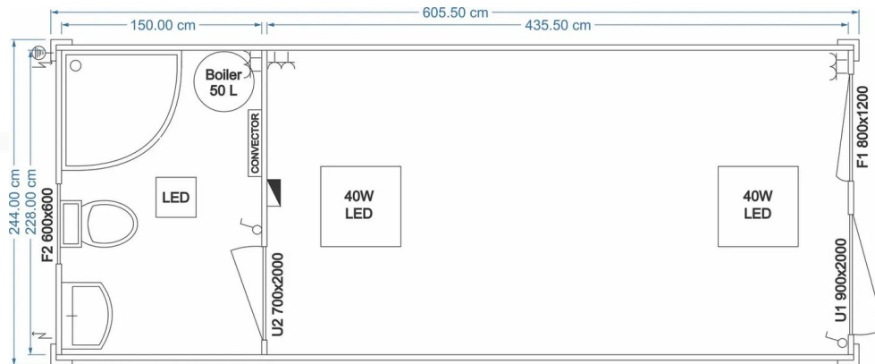
Grundriss (schematisch)
